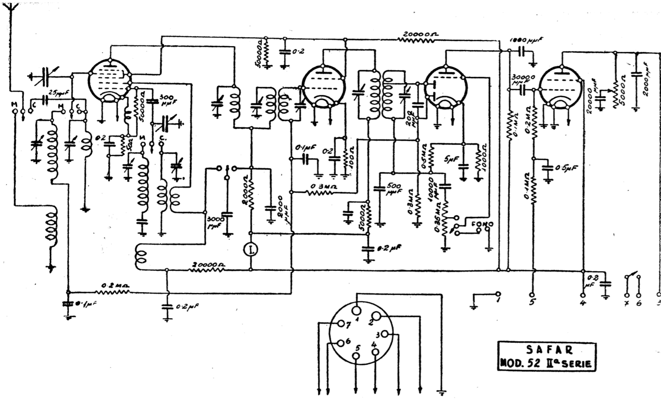
RADIO SAFAR. — Modello « 52 II a serie ». - Produzione 1934. - Media frequenza: 475 kc.
